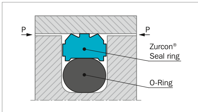
Figure 143: Zurcon® Wynseal
