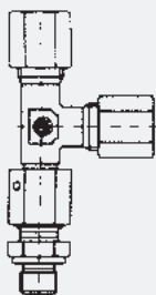
TN 416 - Raccordo combinato orientabile a L con O-Ring - Swivel Barrel Tees with O-Ring seal Pag./Seite 146/147
