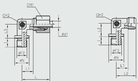
Forma B DIN 3852 Foglio 2 Type B DIN 3852 Part 2
