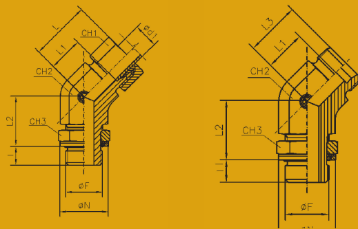
Filettatura: Gas cilindrica Thread: B.S.P. parallel
